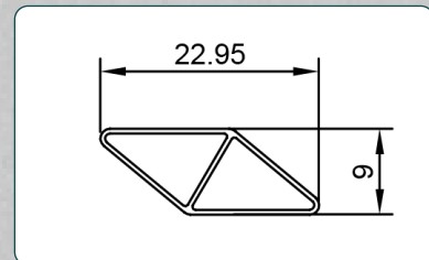
CAB-014
