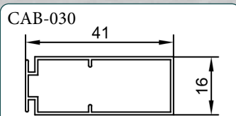
CAB-030 MINI PANEL BOARD
