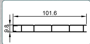
CAB-023
